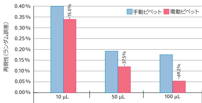
手動ピペットと電動ピペットの再現性比較 (10-100 \mu L容量)
